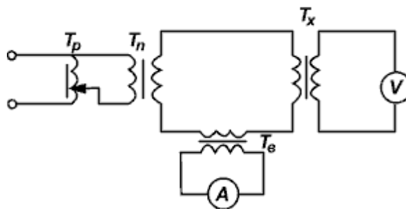
Схема размагничивания трансформатора тока
