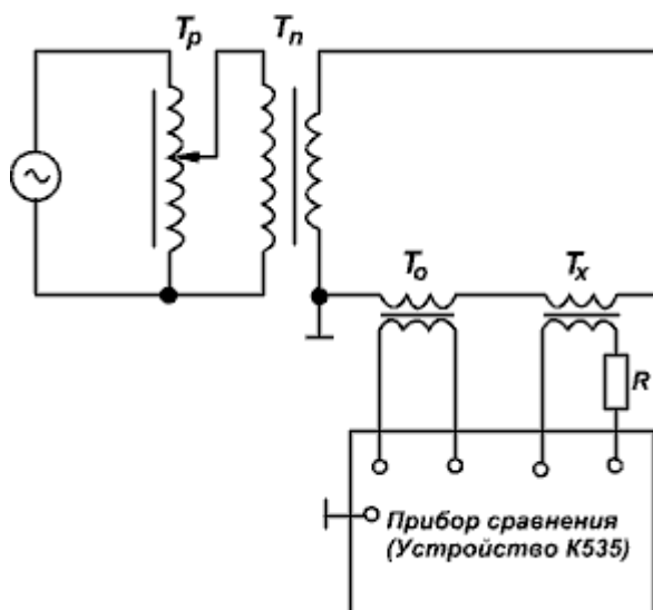
Схема для проверки трансформатора тока дифференциально-нулевым методом с использованием образцового трансформатора тока
